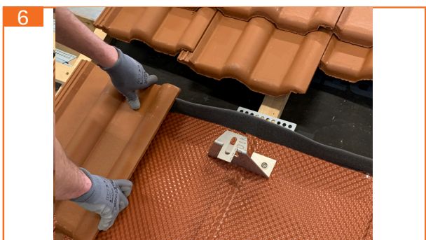
6. geba PV flex einseitig eindecken
