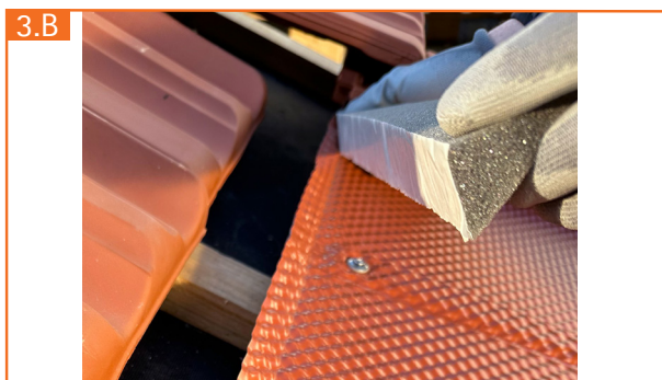
3.B Umlegefalz nach hinten biegen, Kehldichtstreifen auf Umlegefalz kleben
