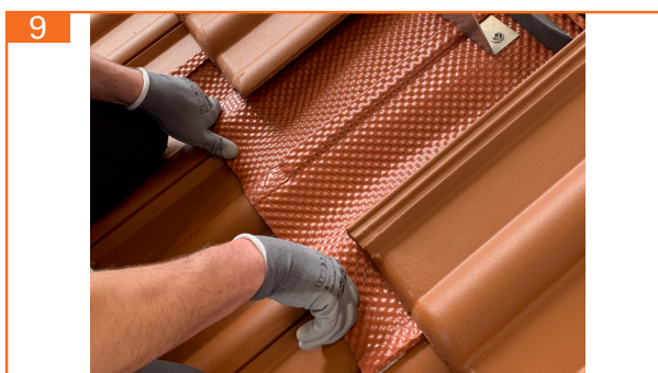
9. geba PV flex an Kontur des Ziegels mittig beginnend nach außen anformen und fest andrücken.
